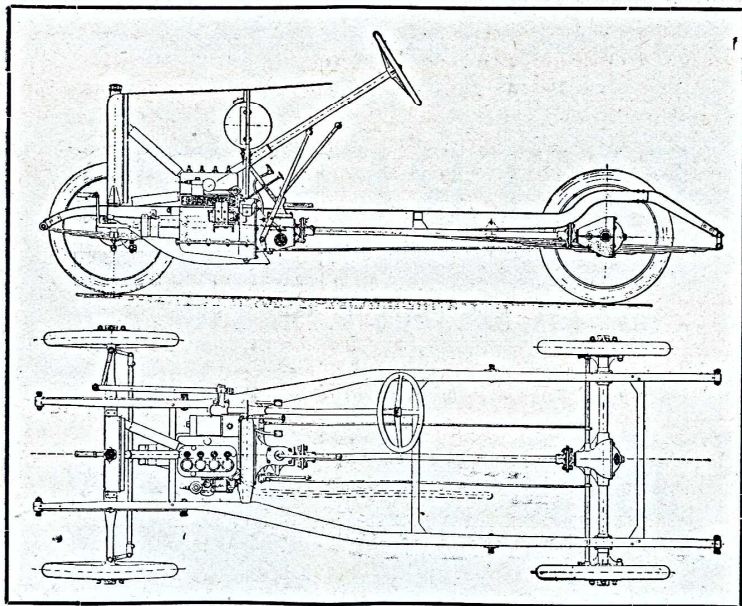
Châssis MATHIS 6 HP, type P (cyclecar)
