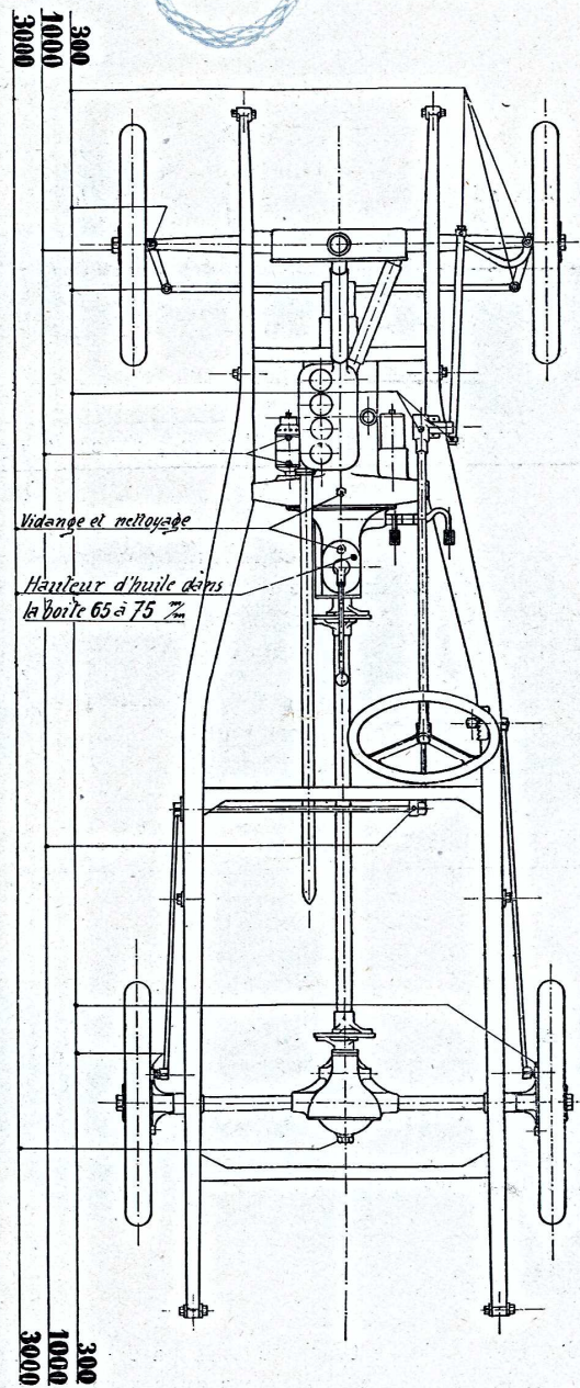
Schéma de graissage du châssis Mathis 6 HP, type P (cyclocar)
