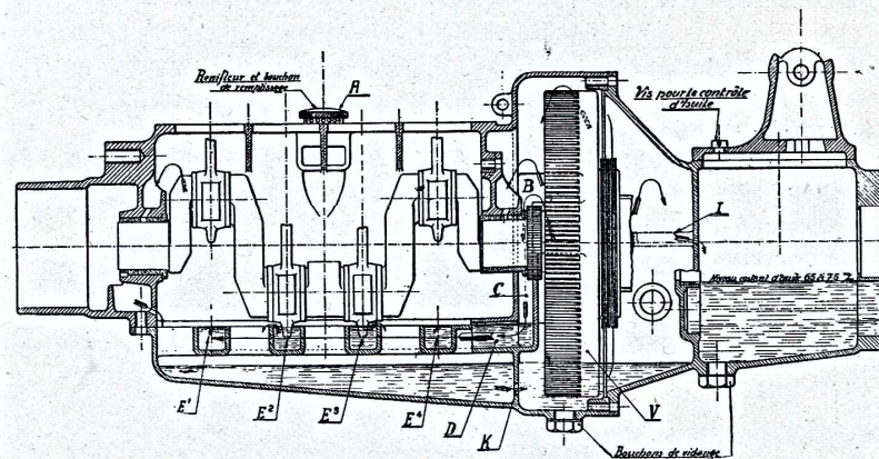
Schéma de graissage du moteur Mathis 6 HP.
