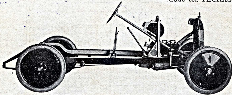
Châssis MATHIS 6 HP avec 5 roues et 4 pneus
